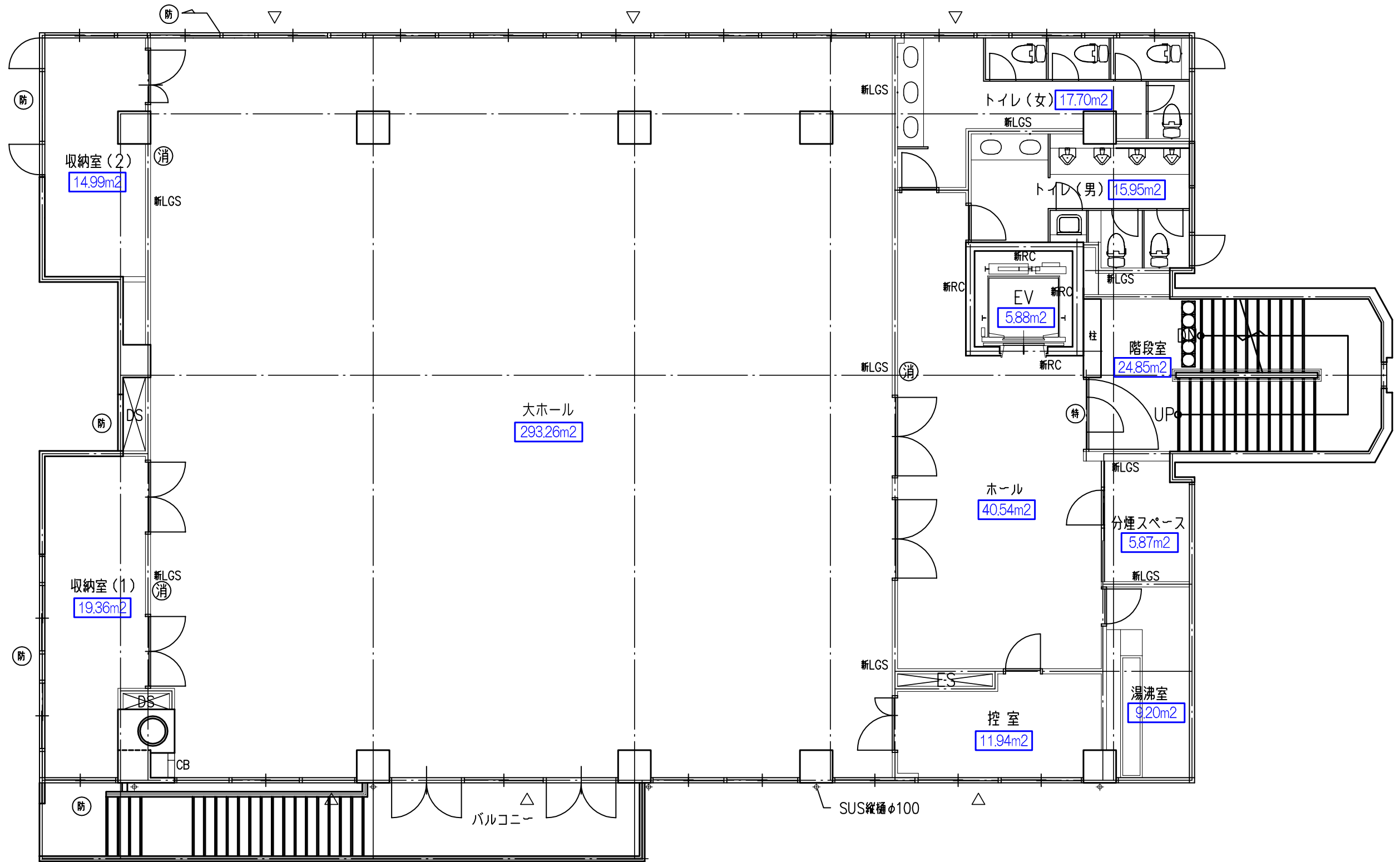
3階平面図
